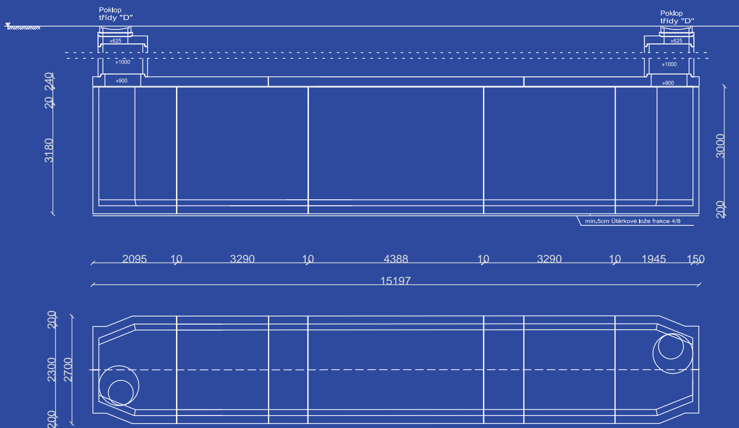
DYWIDAG RB 2700/3180/15200
